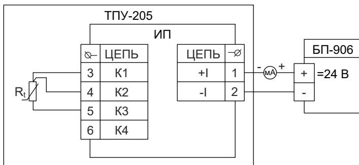
Рисунок А.1 - Трехпроводная схема подключения ТС
